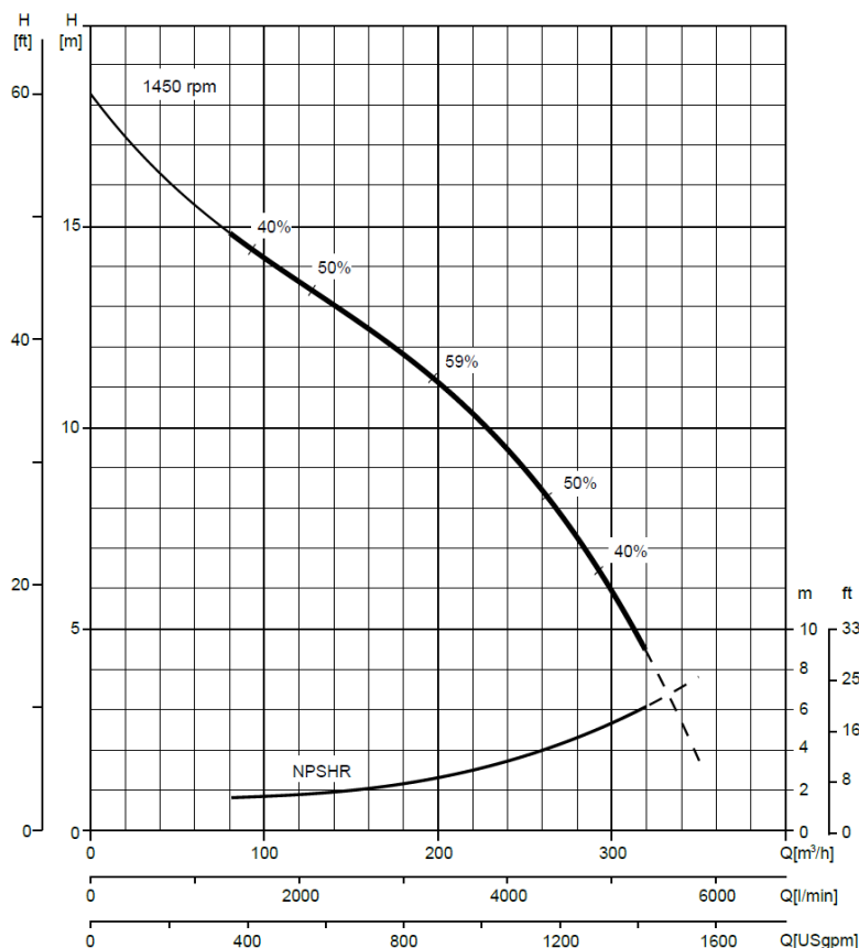
CURVA TECNICA POMPA
